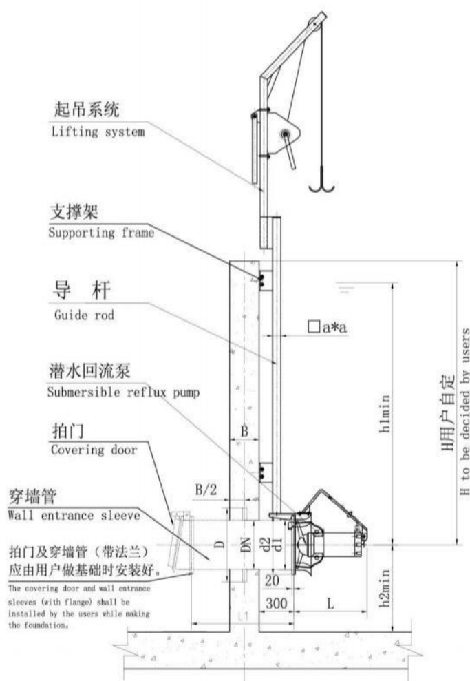
安装示意图
